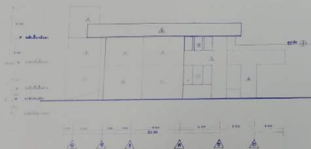
หน้าตัด 2 มาตราส่วน 1:100
