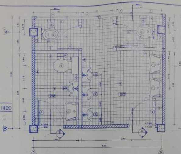
แบบขยายห้องน้ำ-ส่วน 213 1:20
